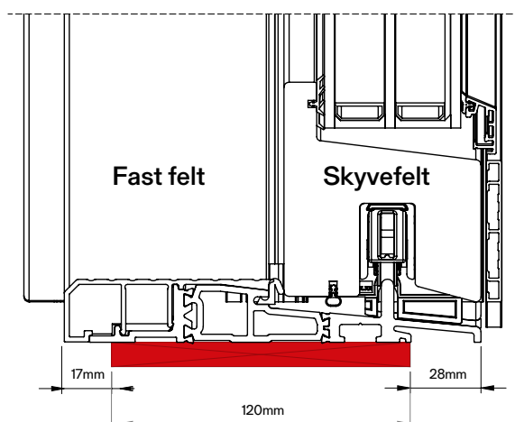
Understøtte, terskel
